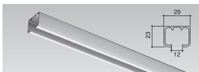
フリータイプ上レール
