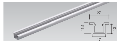
ピボットタイプレール 上/下兼用
